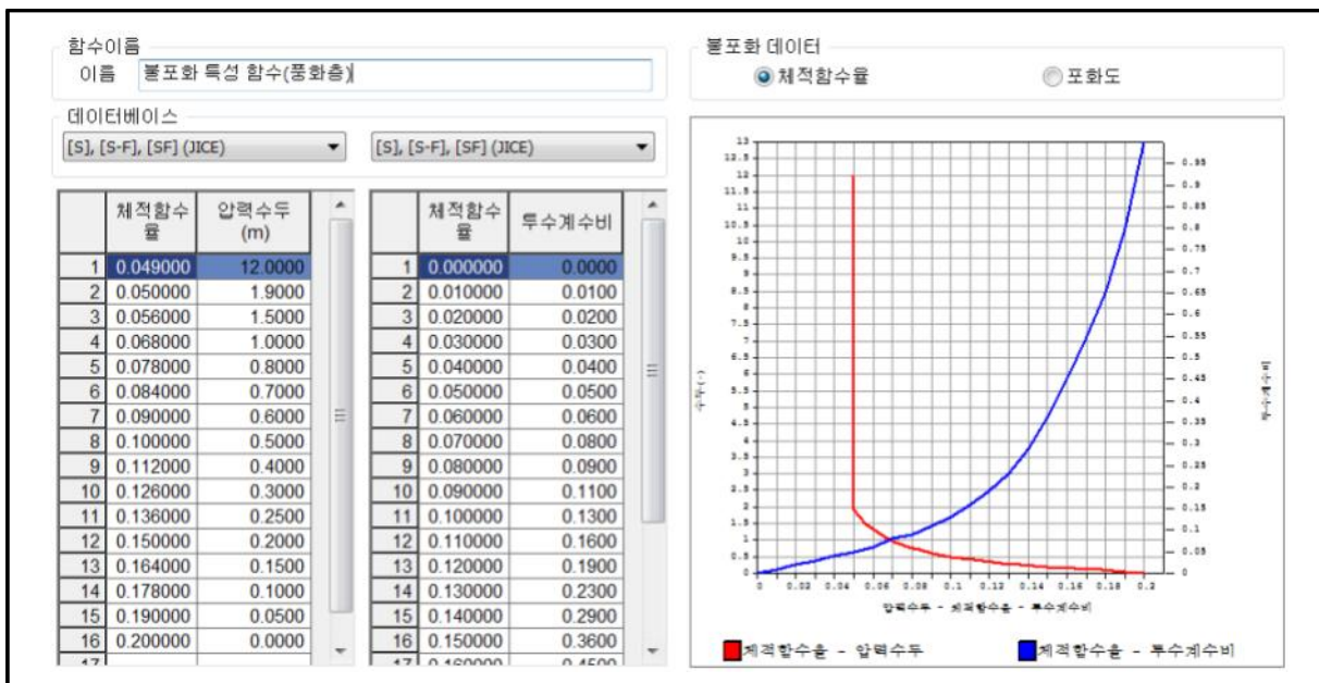
【그림 22.14】 압력수두-채적함수(포화도)-투수계수비 함수
