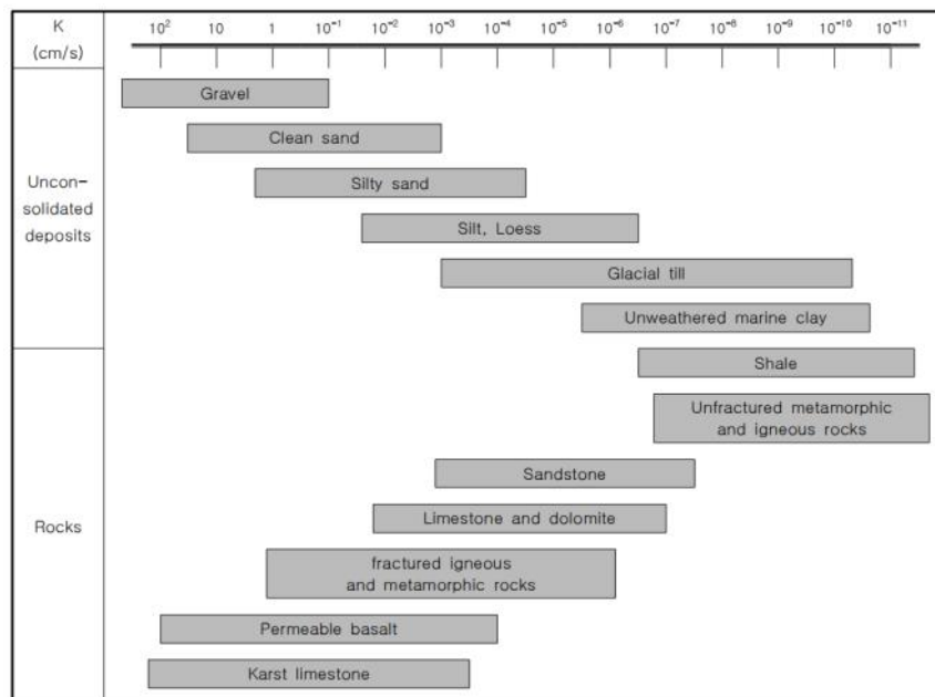
【그림 22.7】 퇴적물 및 암종별 투수계수(Freeze &amp; Cherry, 1979)
