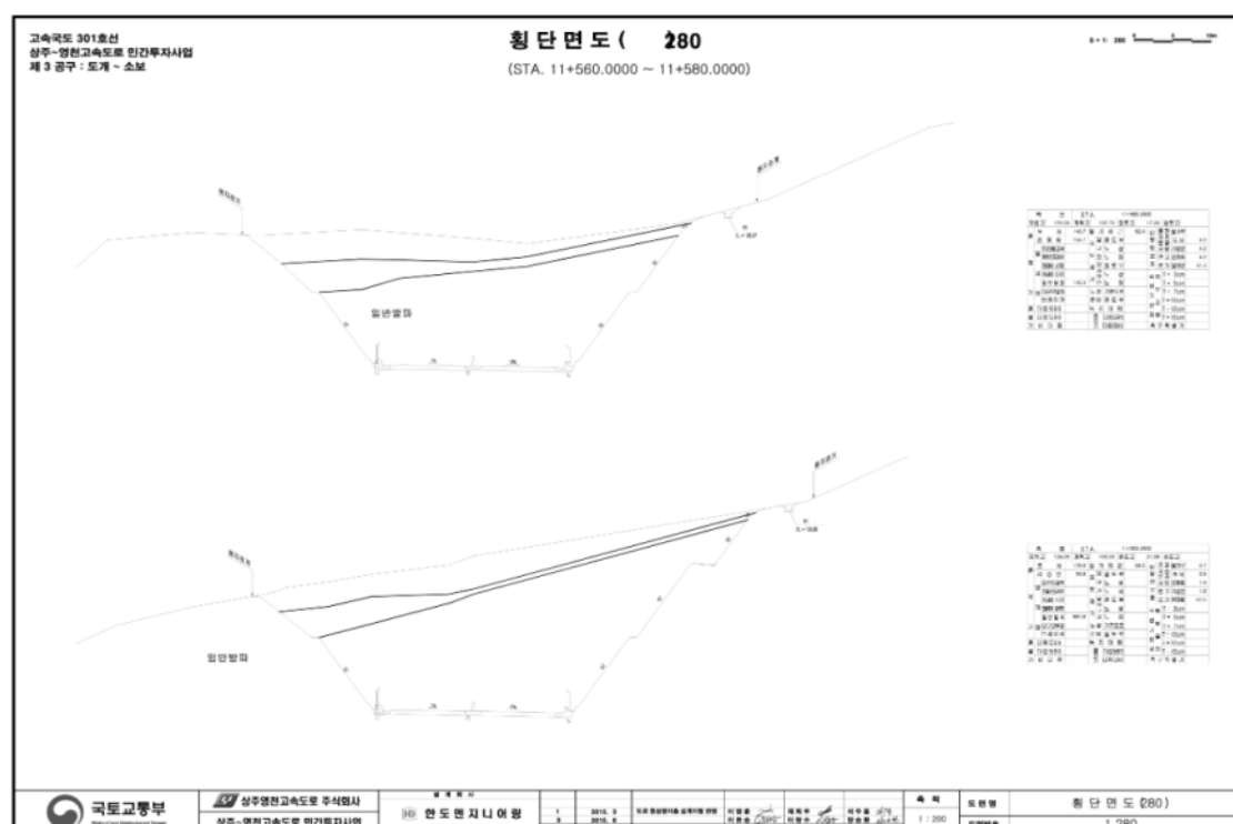
【그림 22.4】 표준횡단면도
